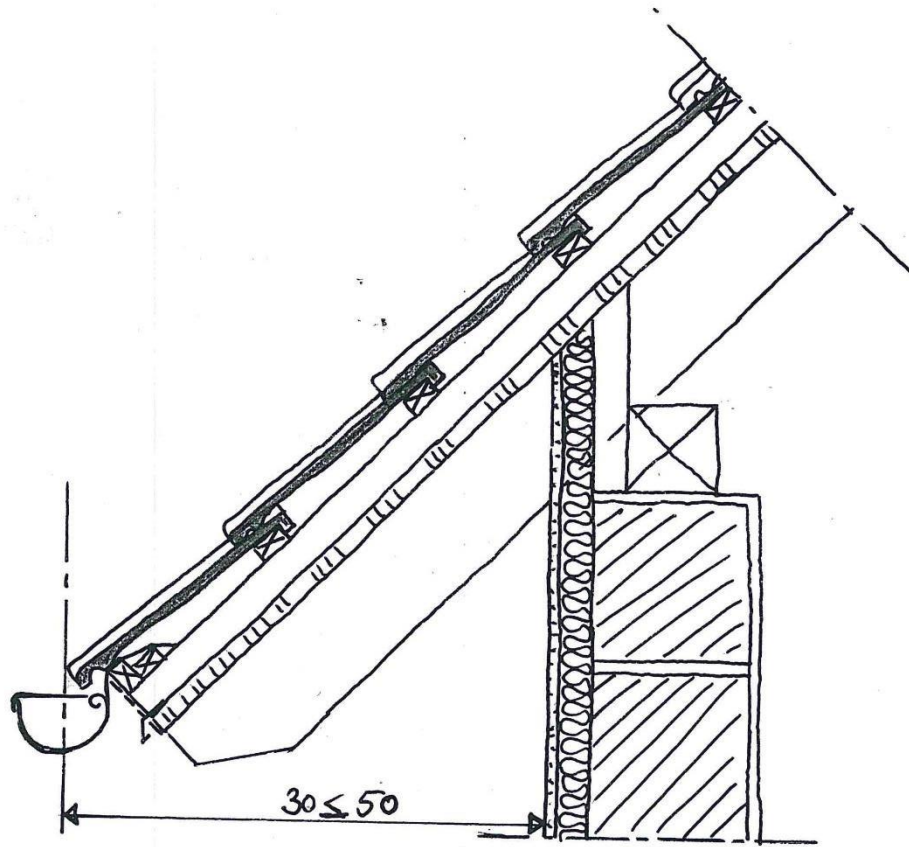
SKIZZE TRAUFE
