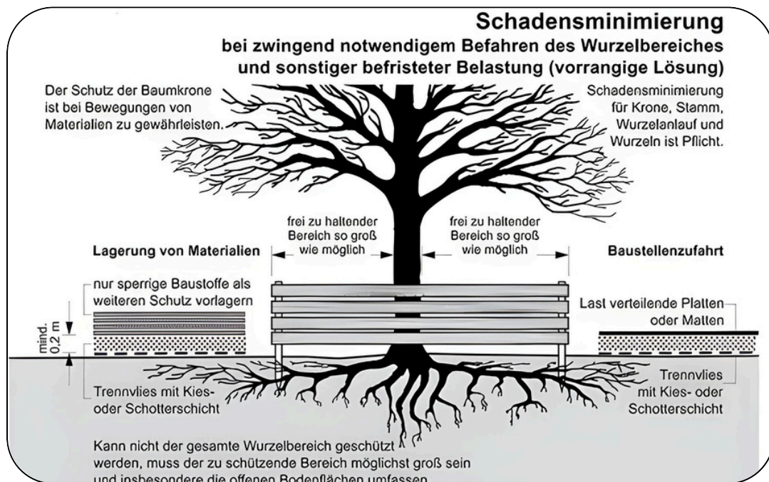
Abbildung 2: Schadensminimierung bei zwingend notwendigem Befahren des Wurzelbereiches und sonstiger befristeter Belastung (vorrangige Lösung) (Dujesiefken, 2025)
