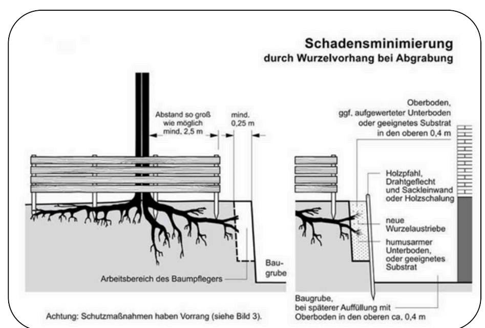
Abbildung 4: Wurzelvorhang bei notwendigen Abgrabungen (Dujesiefken, 2025)
