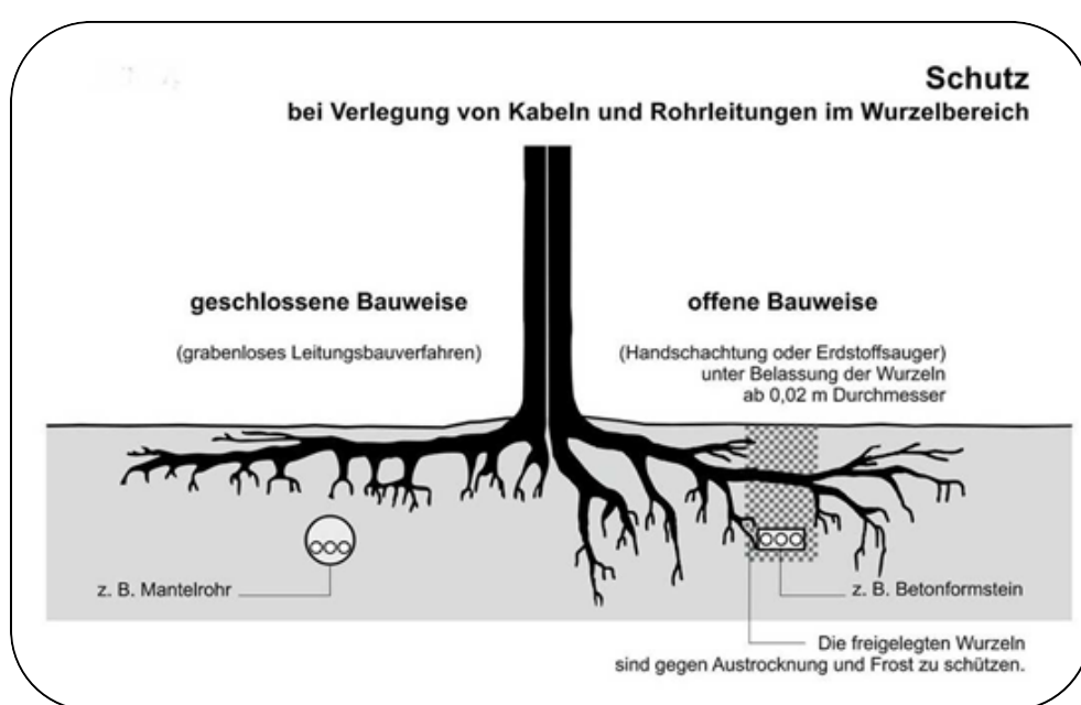
Abbildung 3: Schutz des Baumes bei Verlegung von Kabeln und Rohrleitungen im Wurzelbereich (Dujesiefken, 2025)
